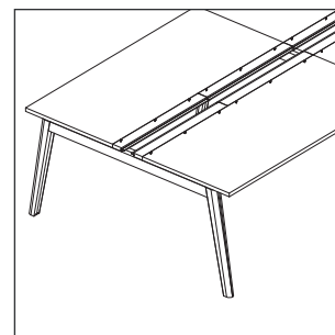
výklop s kartáčem with cable tray with brush
